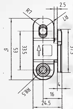
Aufbau der Plattenförderkette mit austauschbaren Förderplatten. Flat top chain with snap-in top design.
