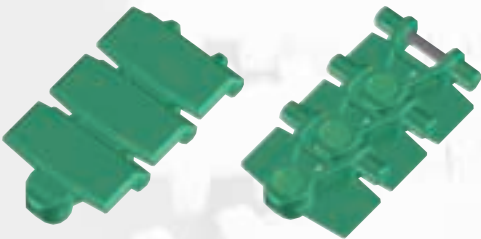
Förderplatte in offener Ausführung Top plate with open top
